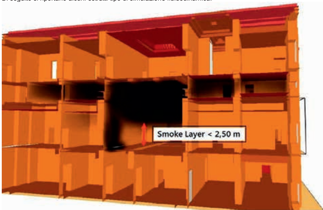
FDS output: simulazione scenario - propagazione del fumo zero exposure (tratta da CFPA - E European Guideline 19:2009)
