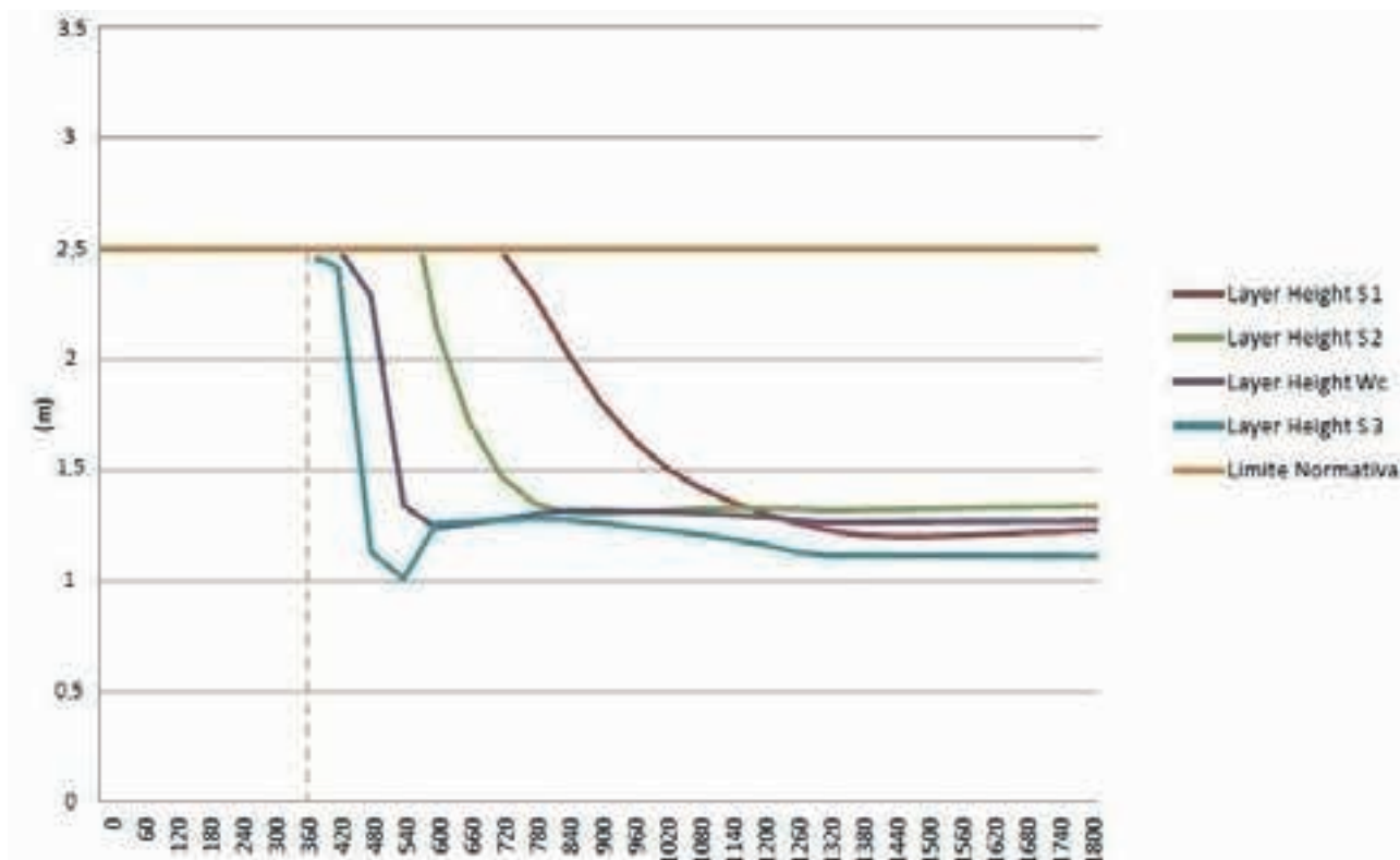
FDS output: simulazione scenario - propagazione del fumo zero exposure (tratta da CFPA - E European Guideline 19:2009)
